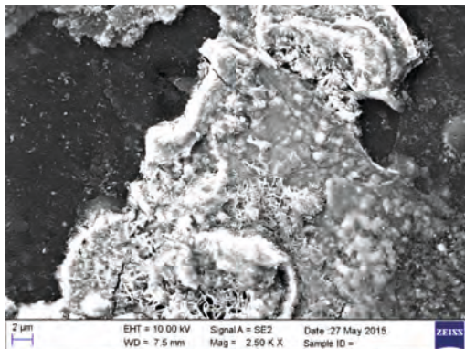
Obr. 13 - Poškozený lak vlivem UV záření.
