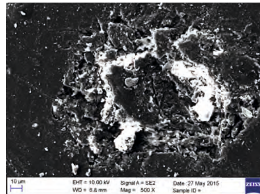
Obr. 15 - Poškození laku od letičiho kamínku
