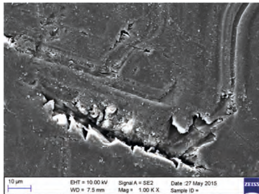
Obr. 14 - Prasklina v laku při 1.000x zvětšení
