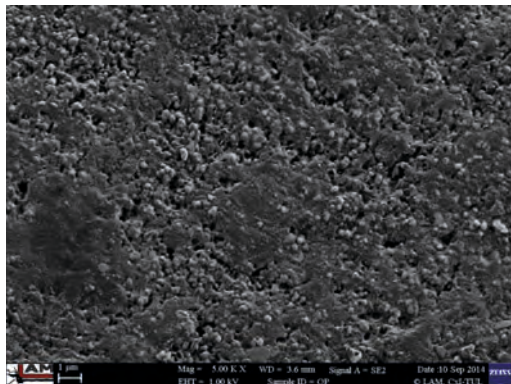
Obr. 10 - Lak neošetřené karoserie zvětšený 5.000x.
